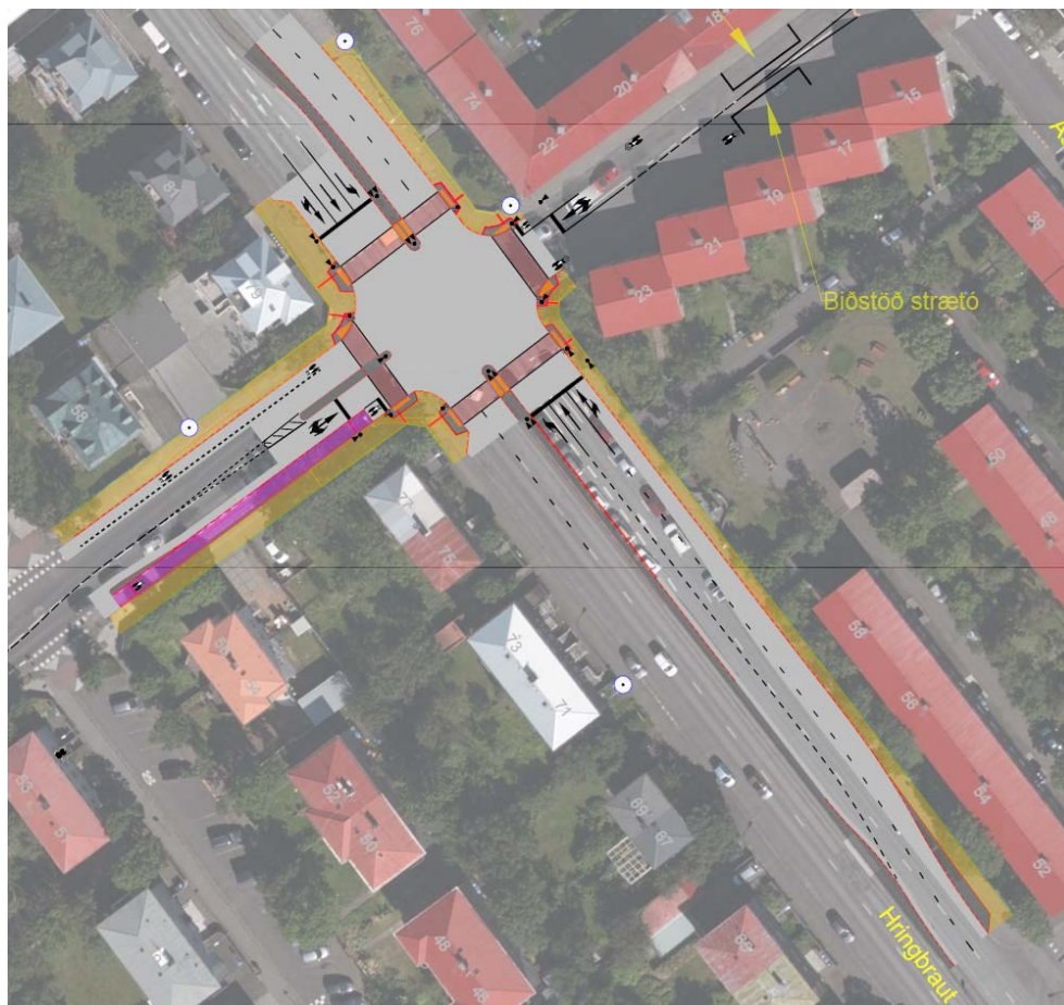
Mynd 1 Forhönnun gatnamóta Hringbrautar og Hofsvallagötu.
